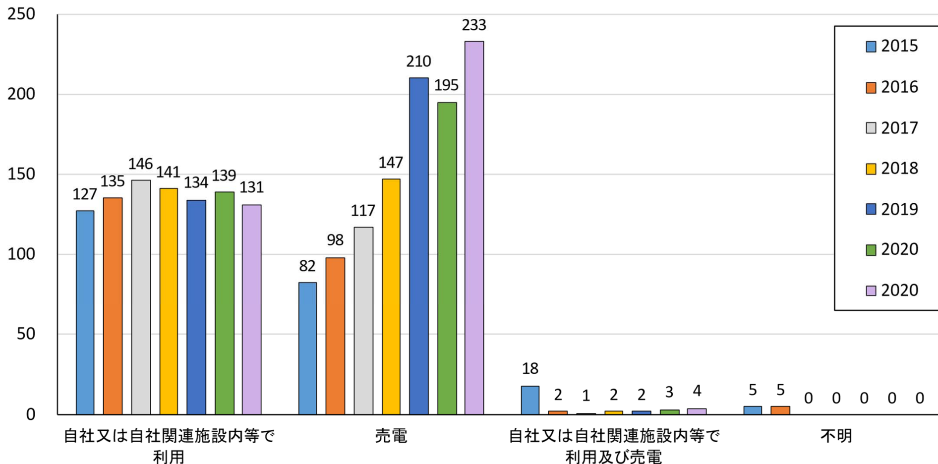
発電機数(基)
