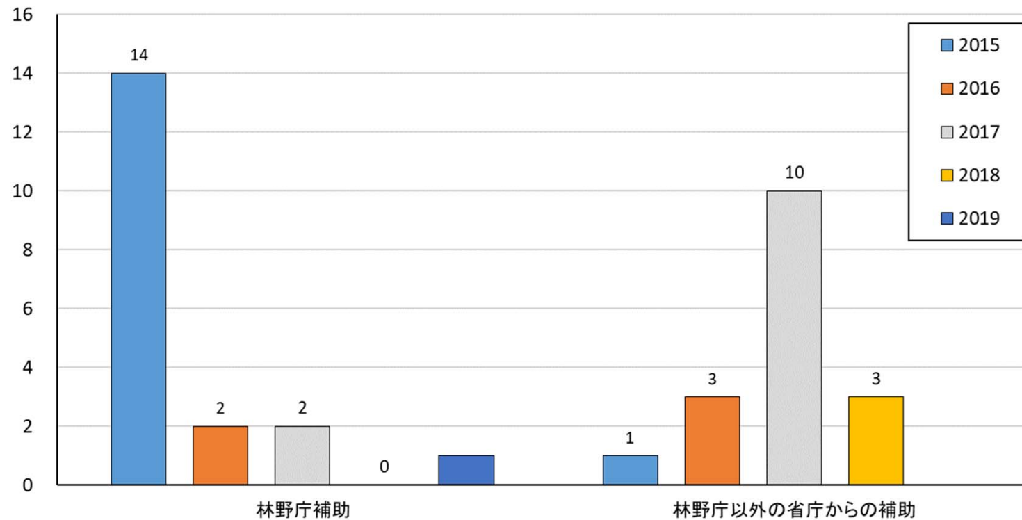
発電機数(基)
