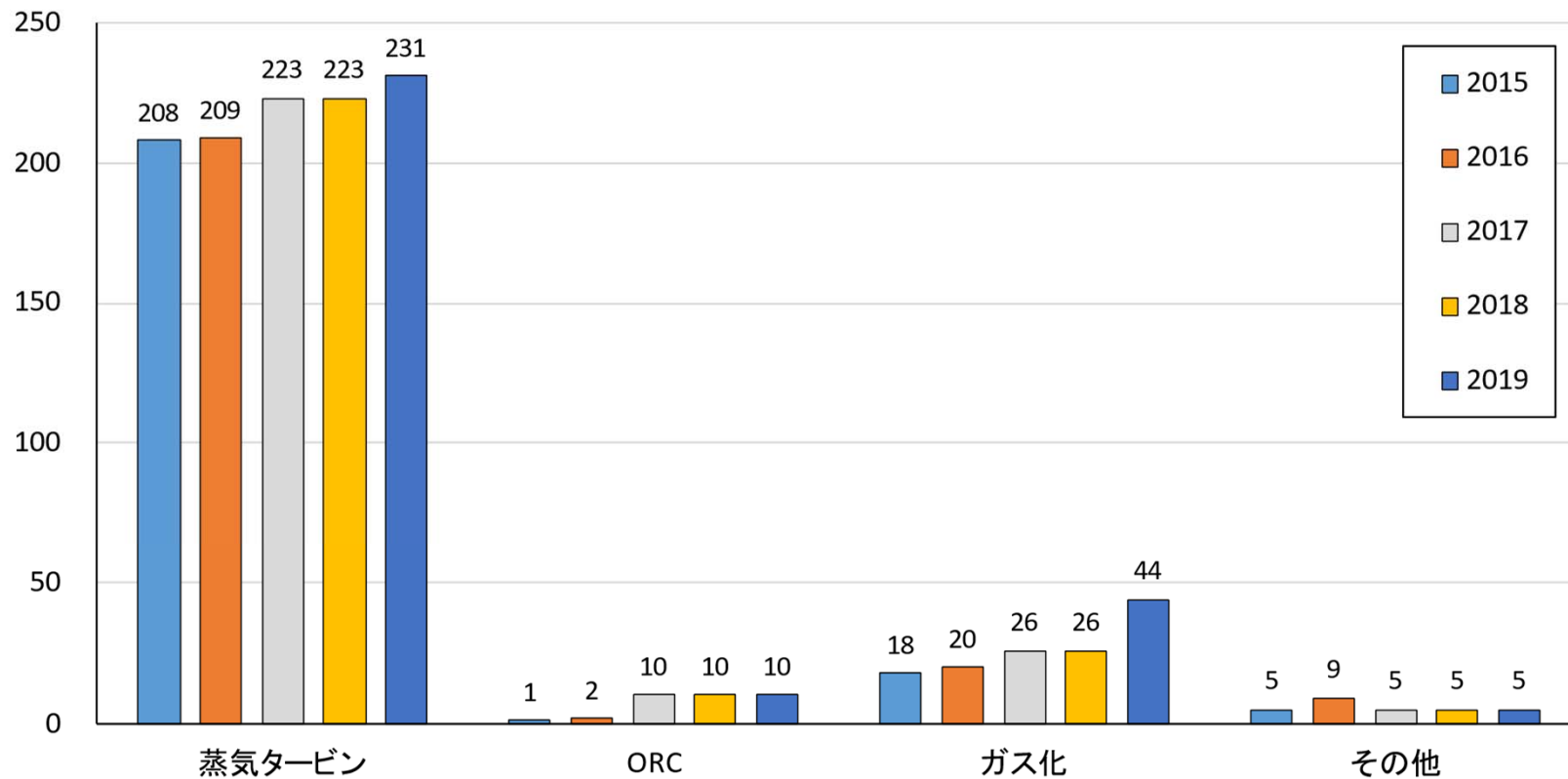
発電機数(基)
